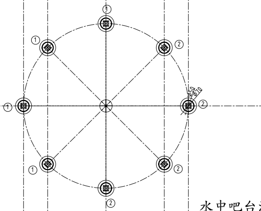
柱位平面圖
